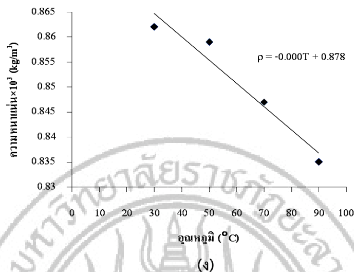
ภาพที่ 28 ค่าความหนาแน่น (ก) น้ำมันถั่วเหลือง (ข) น้ำมันปาล์ม (ค) น้ำมันมะกอก (ง) น้ำมันเครื่อง
