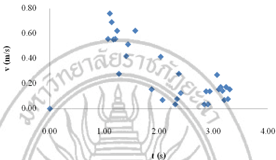
ภาพที่ 27 ความเร็วของการเคลื่อนที่โดยการตกอย่างอิสระของวัตถุภายใต้แรงต้านอากาศ
