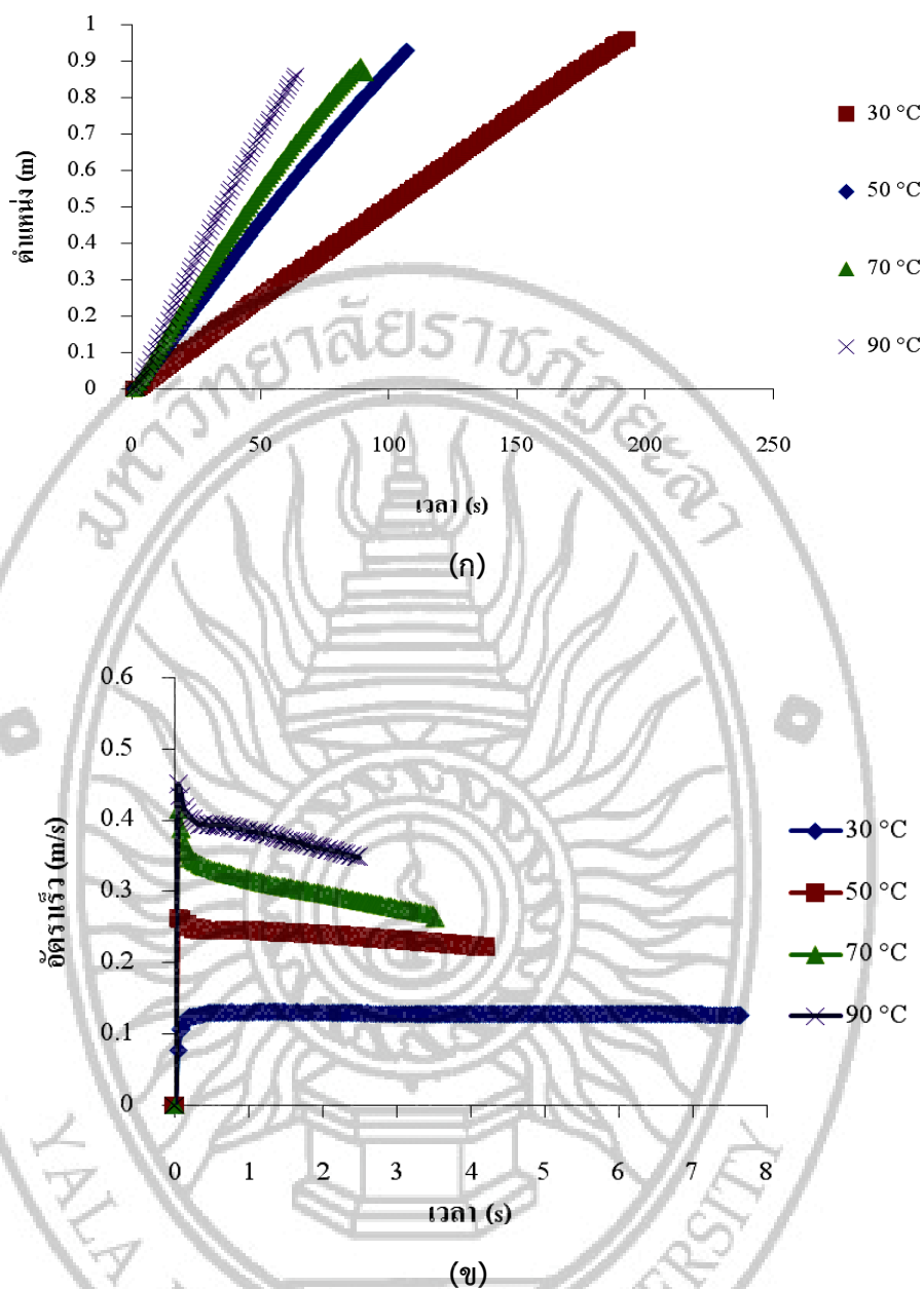
ภาพที่ 32 ผลการวิเคราะห์การเคลื่อนที่ของวัตถุตกผ่านน้ำมันปาล์ม
