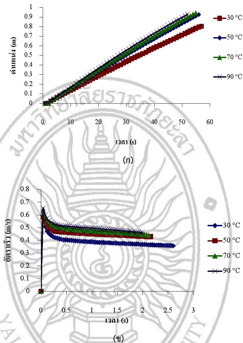
ภาพที่ 31 ผลการวิเคราะห์การเคลื่อนที่ของวัตถุตกผ่านน้ำนํนมะกอก (ก) ตำแหน่งกับเวลา (ข) อัตราเร็วกับเวลา
