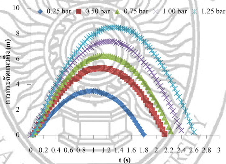
ภาพที่ 41 การกระจัดแนวตั้งของจรวด
