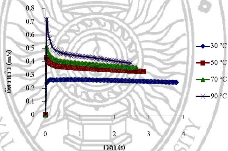
ภาพที่ 30 ผลการวิเคราะห์การเคลื่อนที่ของวัตถุผ่านน้ำมันถั่วเหลือง
