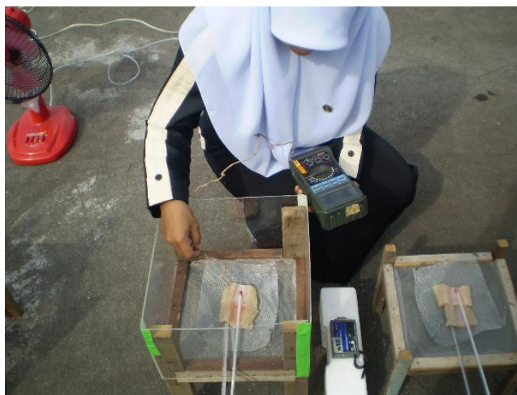
ภาพที่ 3.5 การวัดอุณหภูมิบนผิวหนังตัวปลาได้ผิวหนังและในผิวหนัง
